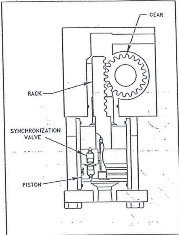
Attuatore invertitore
