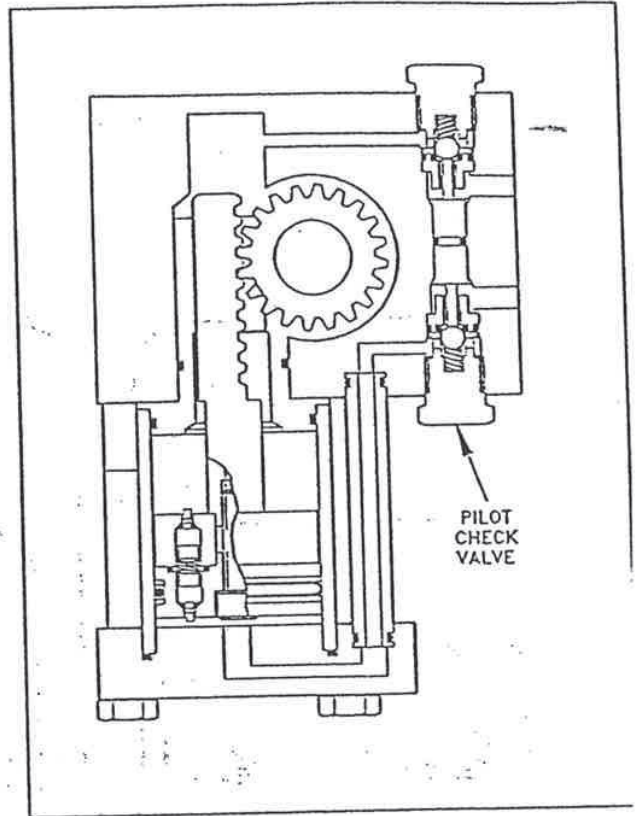
Attuatore acceleratore
