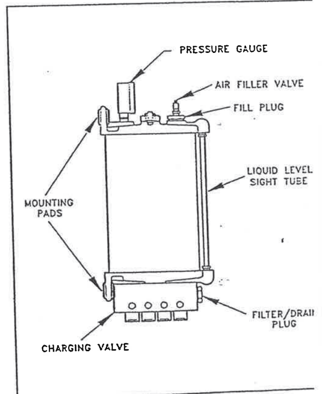
Serbatoio
